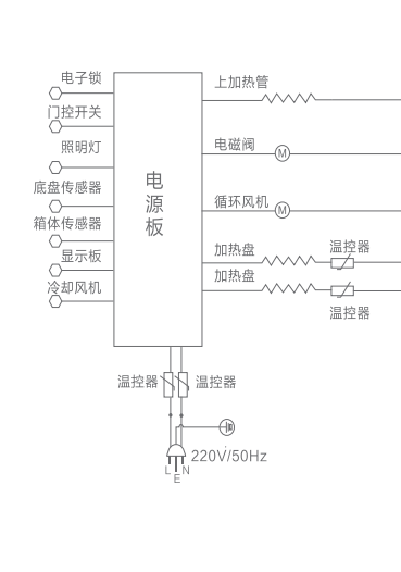
蒸烤箱部分电气原理图
